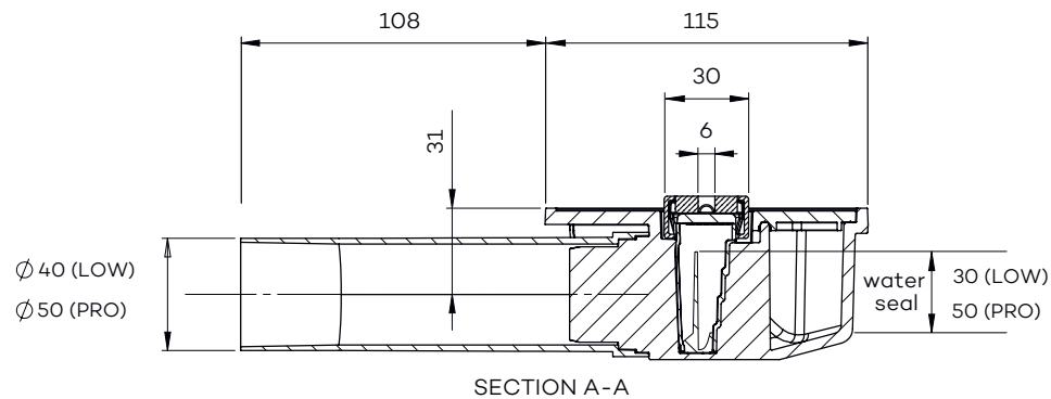
Zijaanzicht
