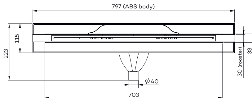
Bovenaanzicht
